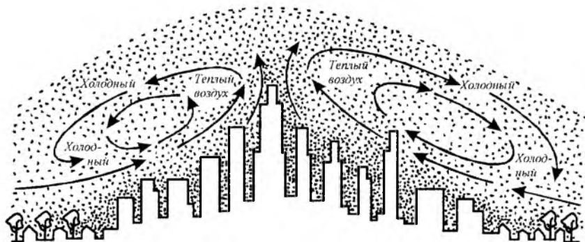
Рис. 9.3. Механизм формирования «купола тепла» над городом
